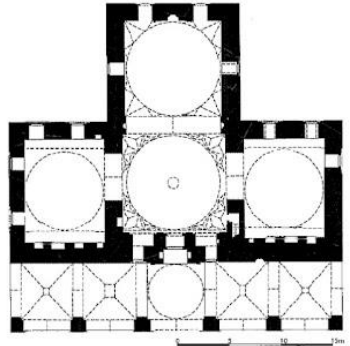
Edirne Muradiye Camii (1426)
