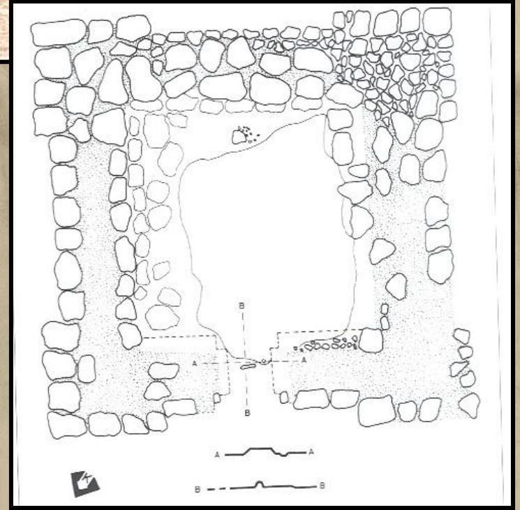
Yukarı Anzaf Tapınağı Taban planı
