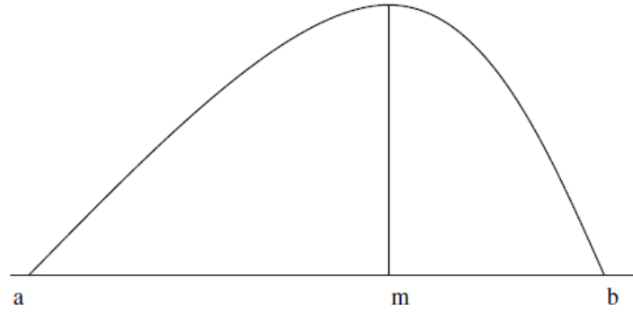
Şekil 17: Sağa Yatkın Beta Dağılımı
