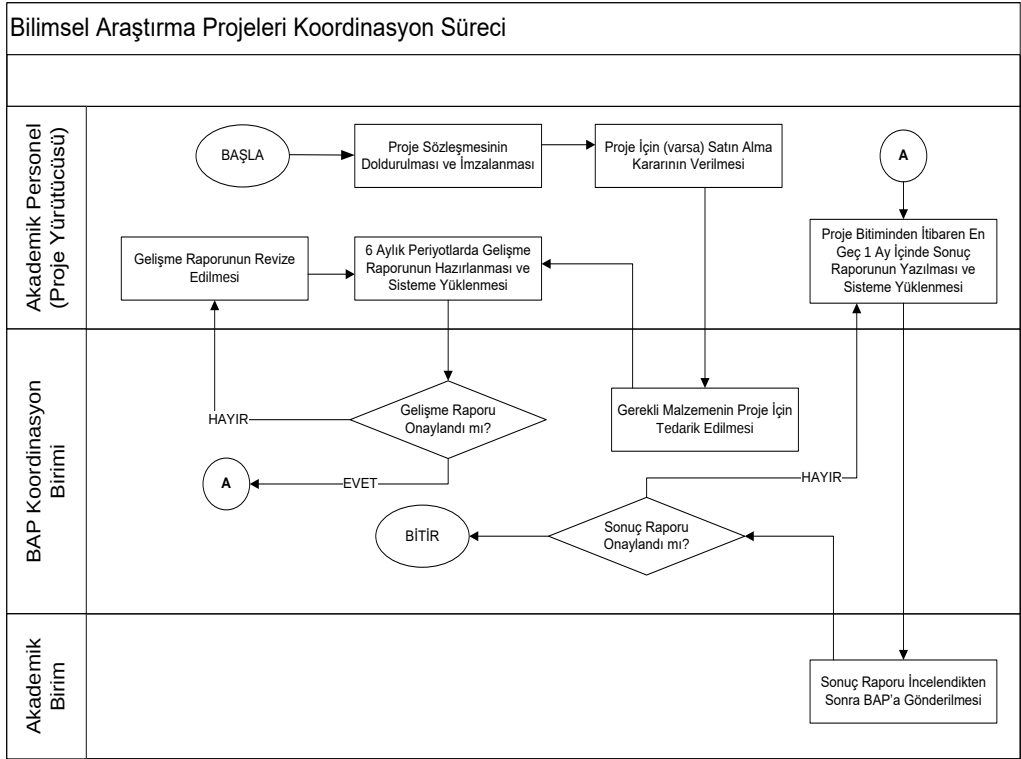
Şekil 2: Bilimsel Araştırma Projeleri Koordinasyon Süreci
