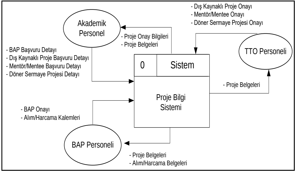
Şekil 3: Bilimsel Araştırma Projeleri Yönetim Bilgi Sistemi Genel Bakış Diyagramı
