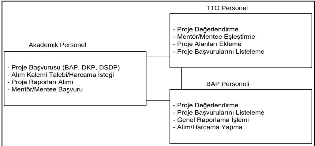
Şekil 4: Bilimsel Araştırma Projeleri Yönetim Bilgi Sistemi Rollere Göre İşlemler
