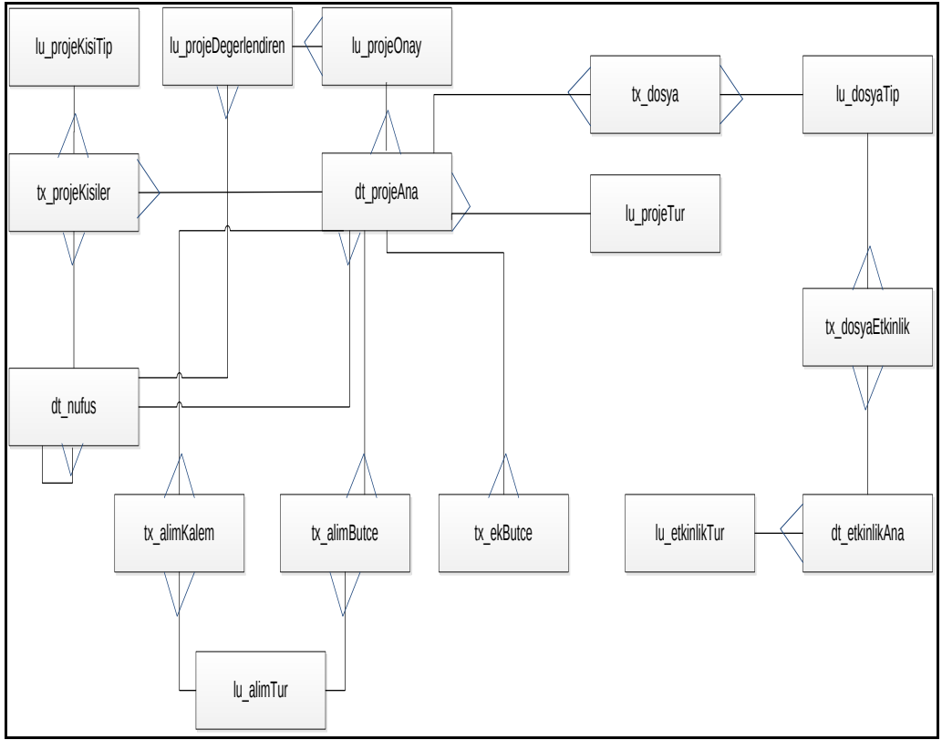
Şekil 5: BAP Veritabanı E-R Diyagramı
