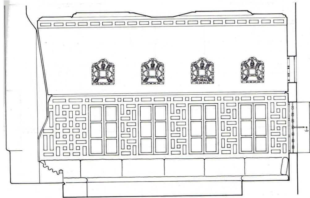
Oda kesiti
