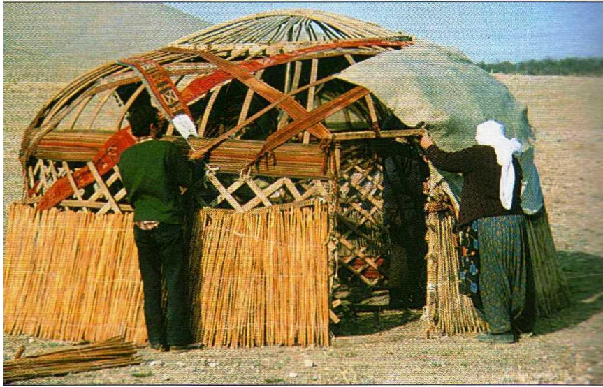
Bir Topak evin hazırlanışı
