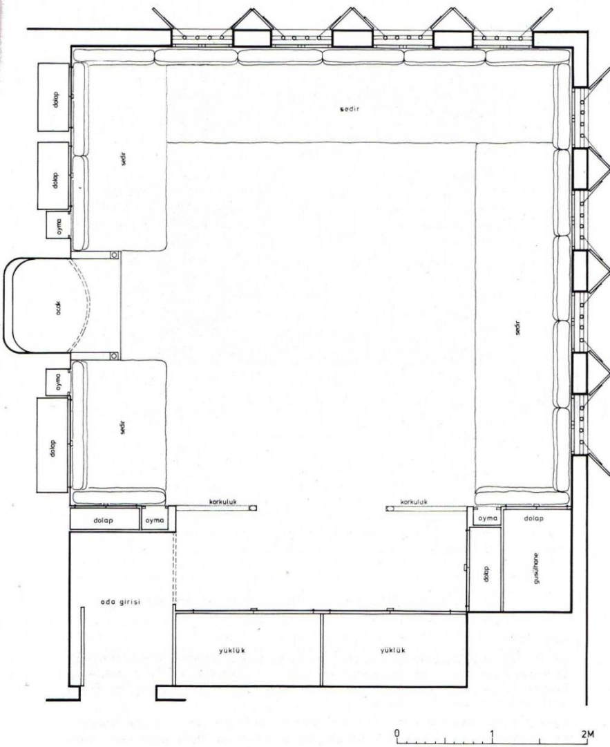
Oda planı
