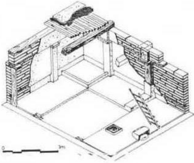
2 Çatalhöyük -Yapı tekniği- Rökonstrüksiyon - M.Ö. 7. Bin (Mellaart'dan)
