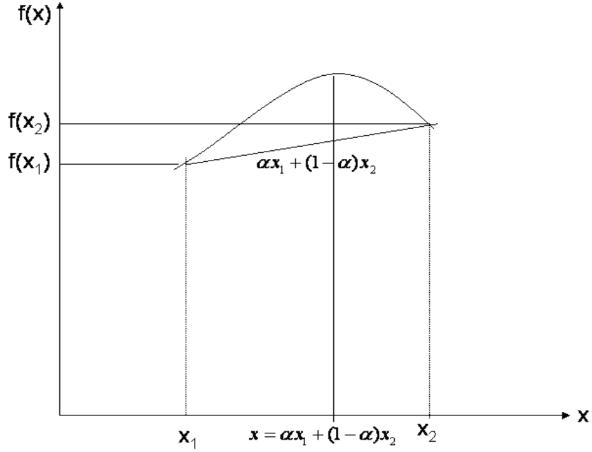
Şekil 2. Konkav fonksiyon
