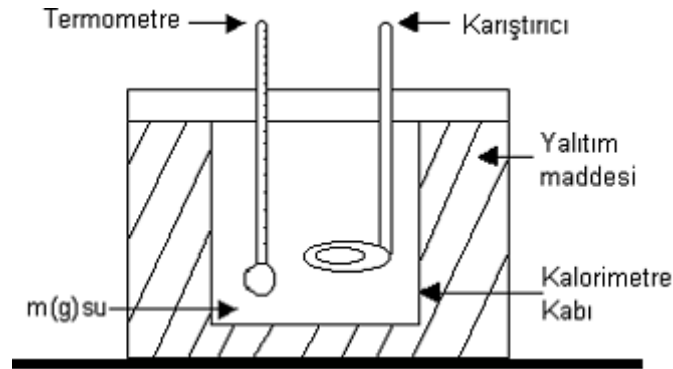
Şekil 8.2. Kalorimetre Kabı
