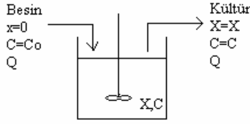
Şekil 2.1. Kermostat
