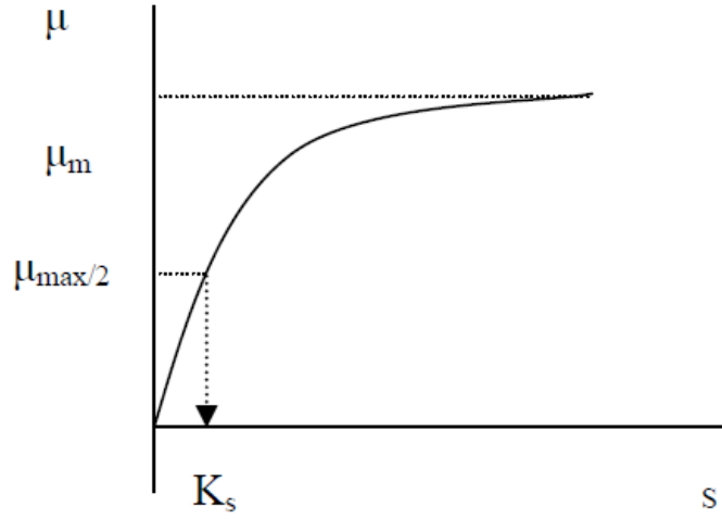
Şekil 2.2. Substrat konsantrasyonunun spesifik büyüme hızı üzerine etkileri.
