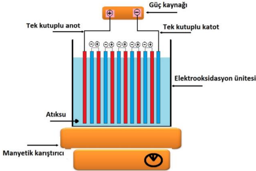
Şekil 5. Tek kutuplu seri bağlı elektrooksidasyon reaktörü
