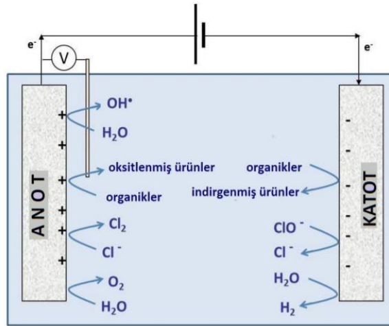
Şekil 2. Elektrokimyasal oksidasyon prosesinde kirliticilerin anot ve katot yüzeyinde parçalanma mekanizması
