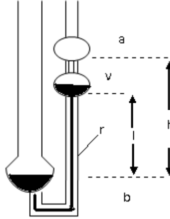
Şekil 3.2. Ostwald viskozimetresi
