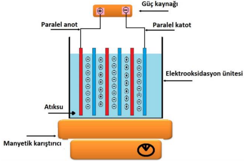
Şekil 6. Çift kutuplu seri bağlı elektrooksidasyon reaktörü
