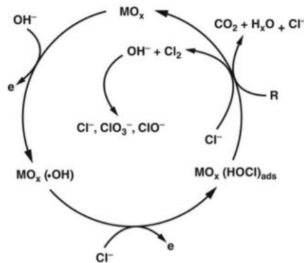
Şekil 4. Organik bileşiklerin ortamda klor bulunması durumunda anot yüzeyinde dolaylı anodik oksidasyonu
