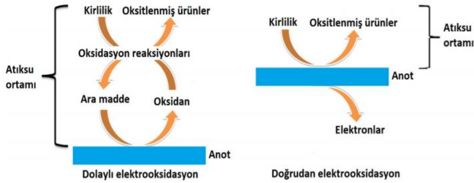
Şekil 1. Elektrokimyasal oksidasyon prosesinde kirliticilerin parçalanması
