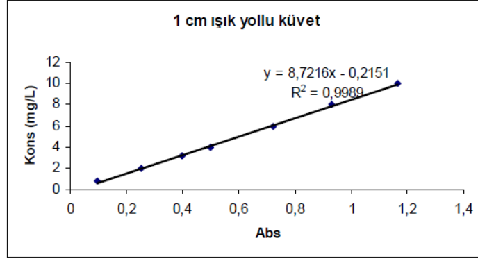
Şekil 7.2. Örnek kalibrasyon eğrisi
