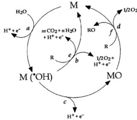
Şekil 3. Organik bileşiklerin aktif (a, c, d ve f reaksiyonları) ve aktif olmayan (a, b ve e reaksiyonları) anot yüzeyinde eş zamanı olarak anodik oksidasyonu
