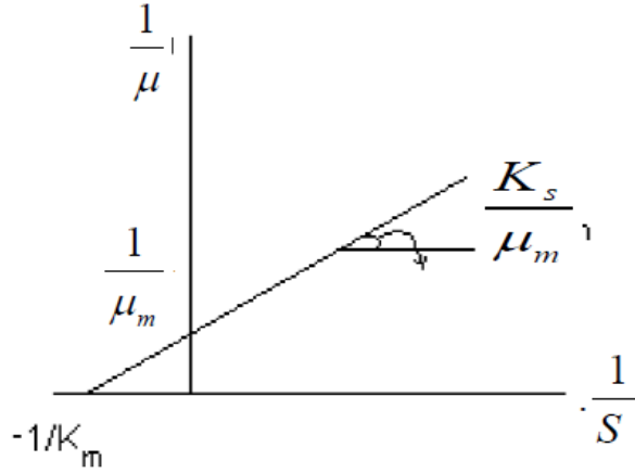
Şekil 2.3. Lineweaver – Burk yaklaşımının grafiksel ifadesi.
